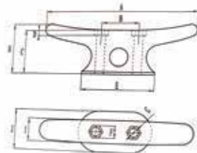
14. Dock Cleat (GM006-92B)
